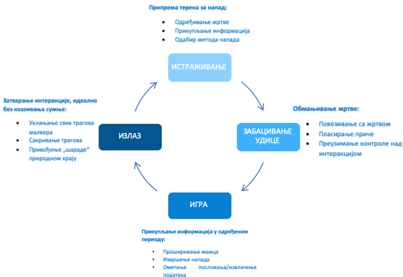
Слика 1. Животни циклус напада социјалног инжењеринга
